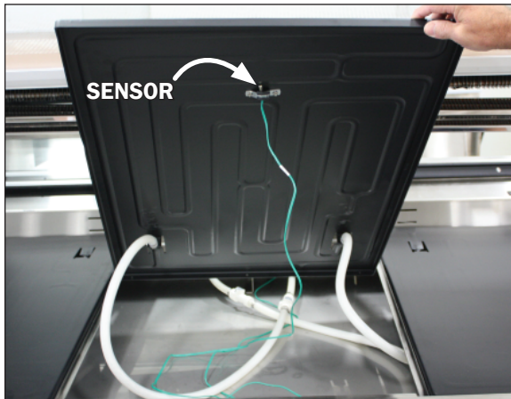
Fig. 3 Coolgenix pan sensor
